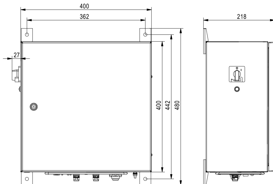
Abb.: Ansichten der Steuereinheit Taurox 900E
