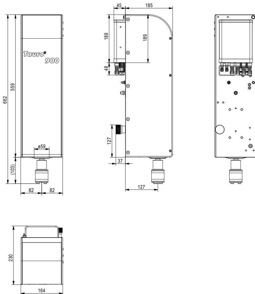
Abb.: Ansichten der Antriebseinheit Taurox 900E
