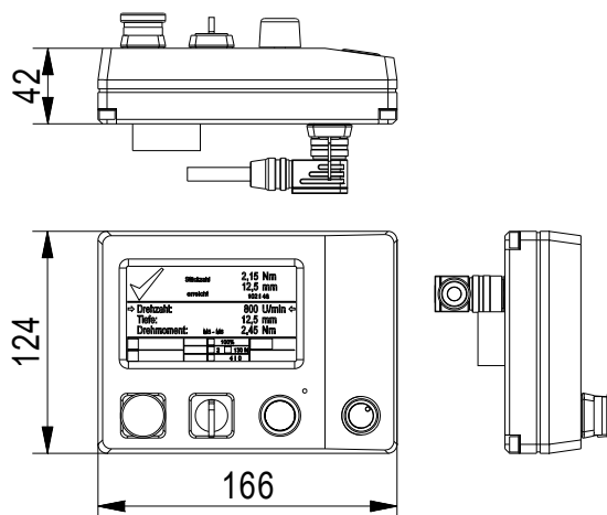
Abb.: Ansichten der Bedieneinheit Taurox 900E
