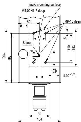
Abb.: Flanschmaße der Antriebseinheit Taurox 900E
